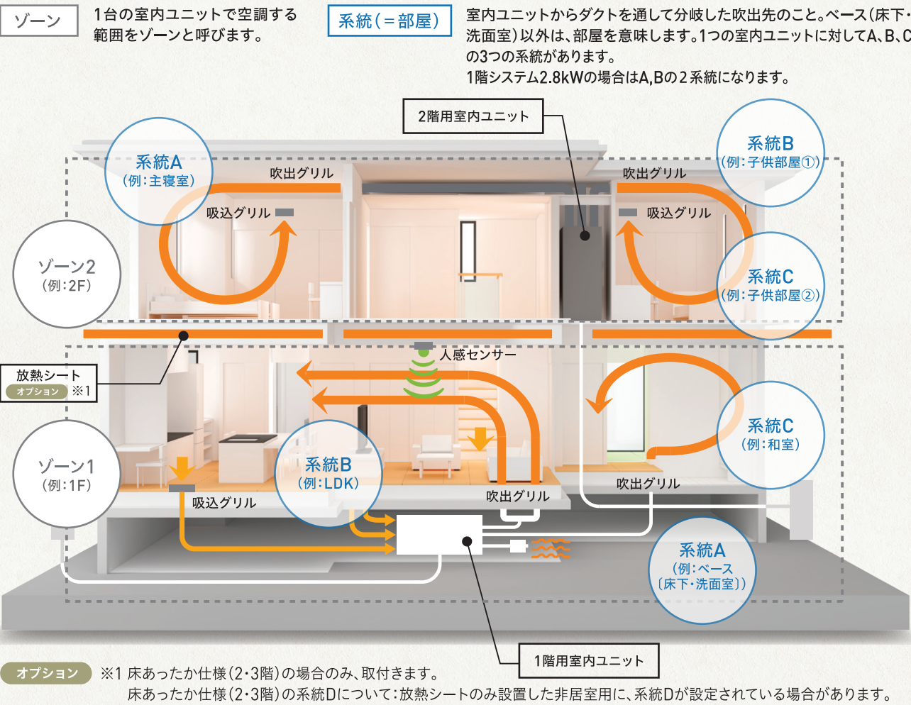
全体構成図
